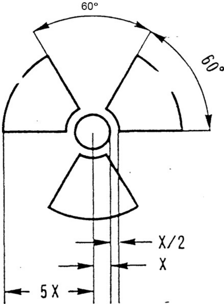
Рисунок 1. Основной знак радиационной опасности в виде трилистника, пропорции которого определяются по центральной окружности радиуса X . Минимальная допустимая величина X равна 4 мм.
